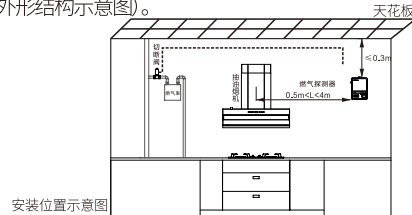
安装位置示意图
